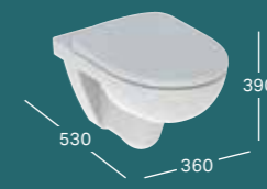
PAKET GEBERIT SELNOVA, B 360 / H 390 / T 530 konzolna WC školjka, djelomično zatvorene forme, Rimfree® WC sjedalo s poklopcem, funkcija SoftClose, funkcija QuickRelease
